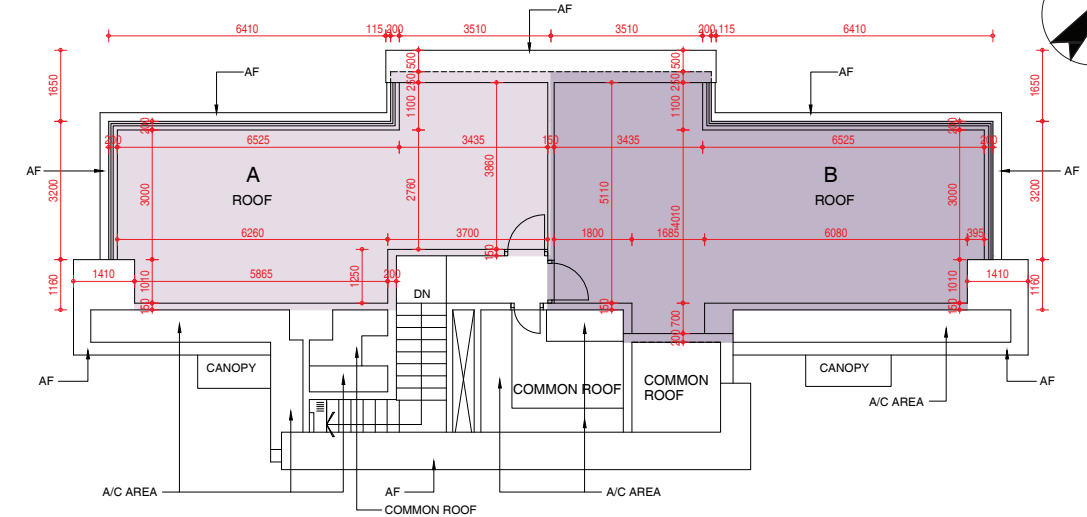
Roof Floor Plan 天台樓面平面圖
