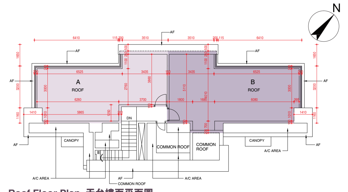
Roof Floor Plan 天台樓面平面圖
